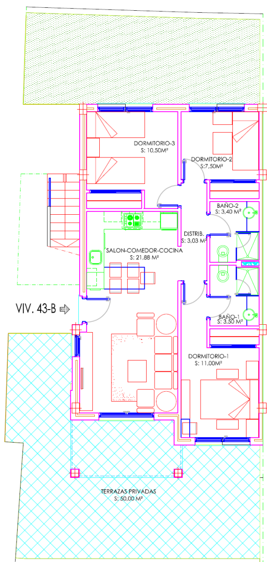
PLANTA BAJA
